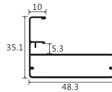
A-8AF 粗鋁框【有把手】
