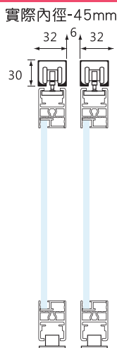
一般懸吊鋁門側剖圖
