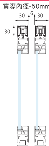
緩衝懸吊鋁門側剖圖
