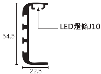
下櫃用無把手設計-C型
