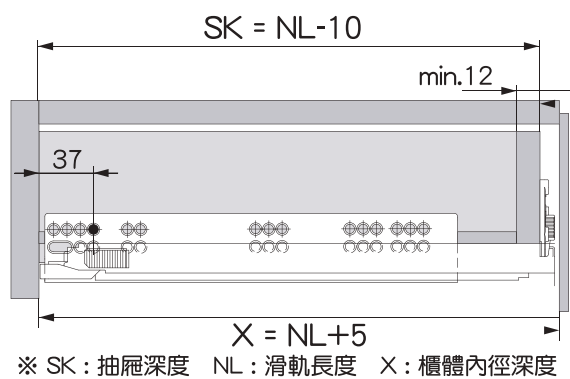
外抽尺寸圖
