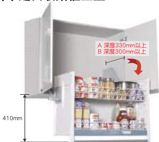
緩衝昇降收納櫃 (三段調整載重)
