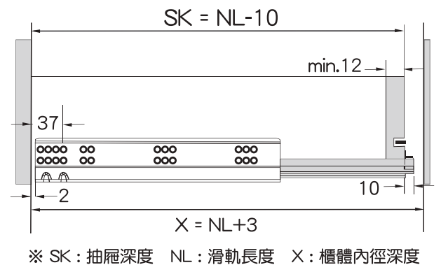
外抽尺寸圖
