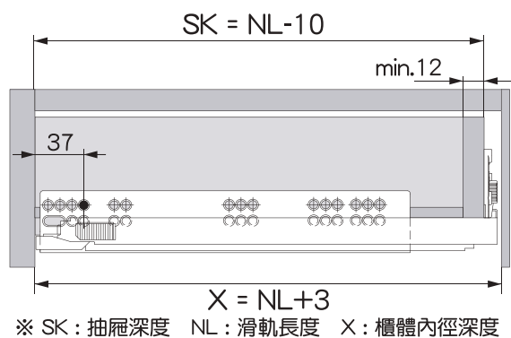
外抽尺寸圖
