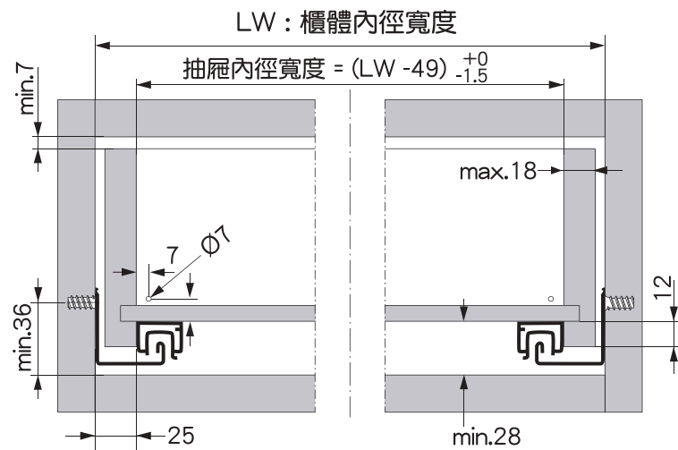
抽屜組裝位置圖
